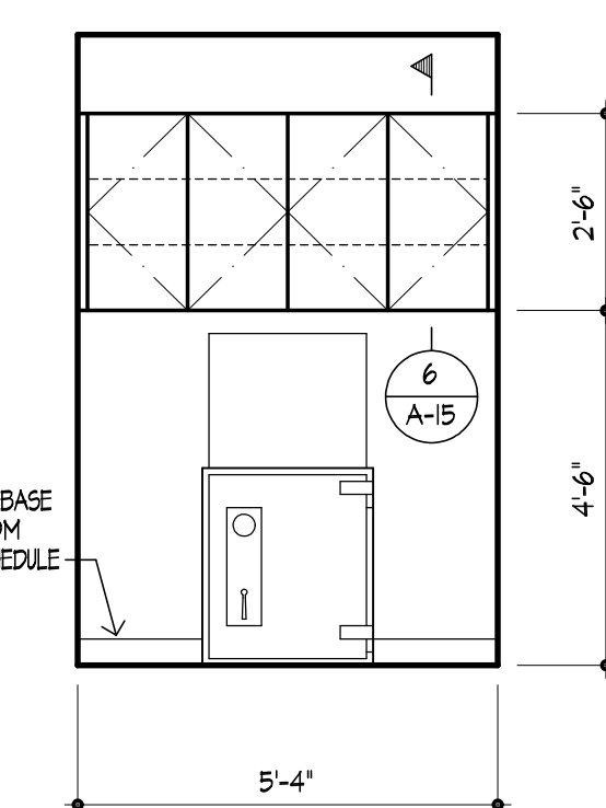
10 ELEV NIGHT DEPOSIT 117
